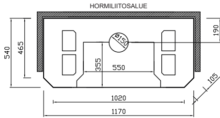
HILDA 120 SUORAMALLI EI NURKKAMALLIA
