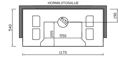
FIONA 120 SUORAMALLI EI NURKKAMALLIA
