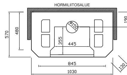
SANDRA SUORAMALLI EI NURKKAMALLIA
