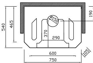
HILDA 75, SANTERI 75, VALKEA 75 SUORAMALLI
