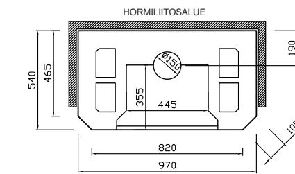
SANTERI 100, HILDA 100, VALKEA 100 SUORAMALLI EI NURKKAMALLIA
