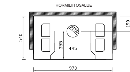
FIONA 100 SUORAMALLI EI NURKKAMALLIA
