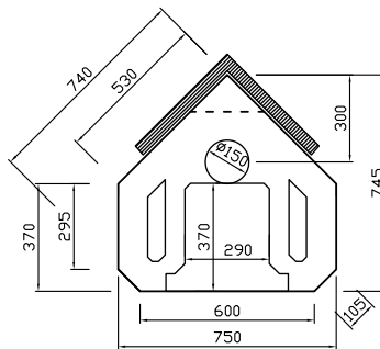
HILDA 75, SANTERI 75, VALKEA 75 NURKKAMALLI
